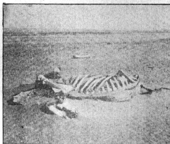
Fig. 9 — Alusão da revista brasileira "Planeta" (nr. 168, Set. 1986), ao avanço da desertificação terrestre, na base de 5 km cada ano.
