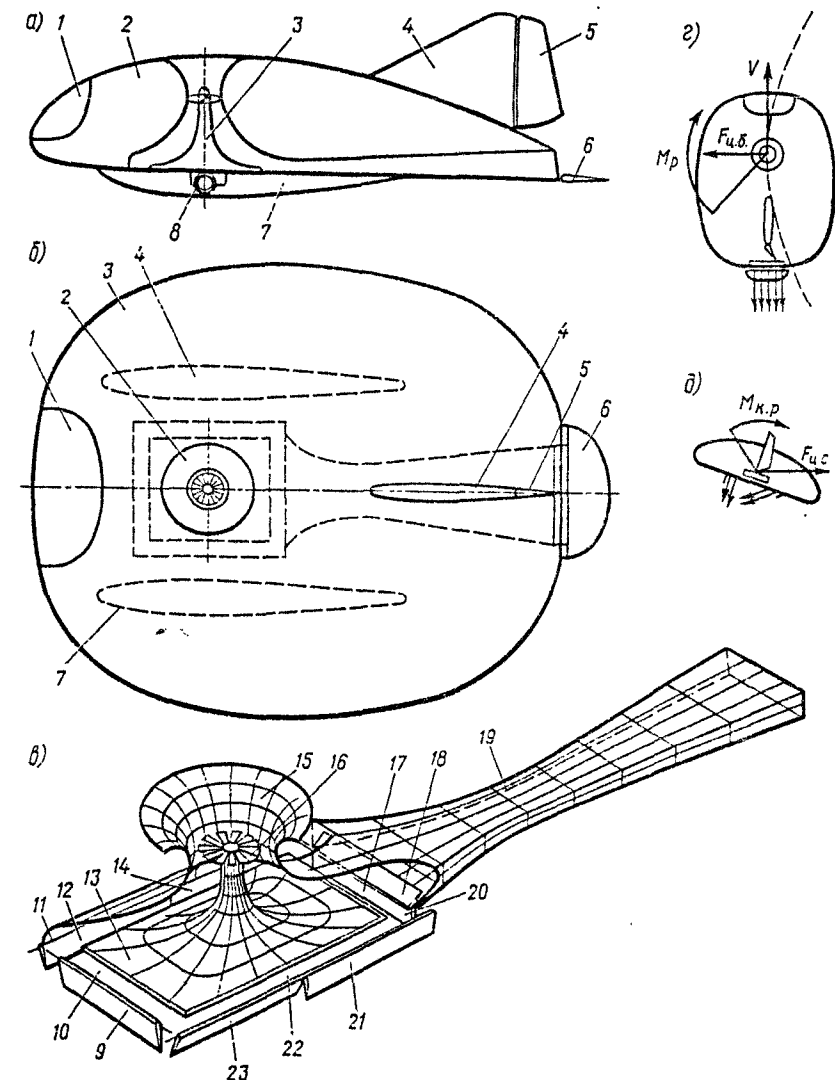
Рис. 255. Гибридный дирижабль: а — вид сбоку; б — вид сверху; в — схема воздухометного дирижабля; г — схема сил и моментов, действующих на аппарат при полете по криволинейной траектории; д — то же, вид сзади; 1 — кабина; 2 — корпус; 3 — воздухометный движитель; 4 — киль; 5 — руль направления; 6 — руль высоты; 7 — емкость; 8 — двигатель; 9, 11, 14, 18, 20, 21, 23 — створки; 10, 12, 17, 22 — щели; 13 — ресивер; 15 — диффузор; 16 — вентилятор; 19 — воздуховод
