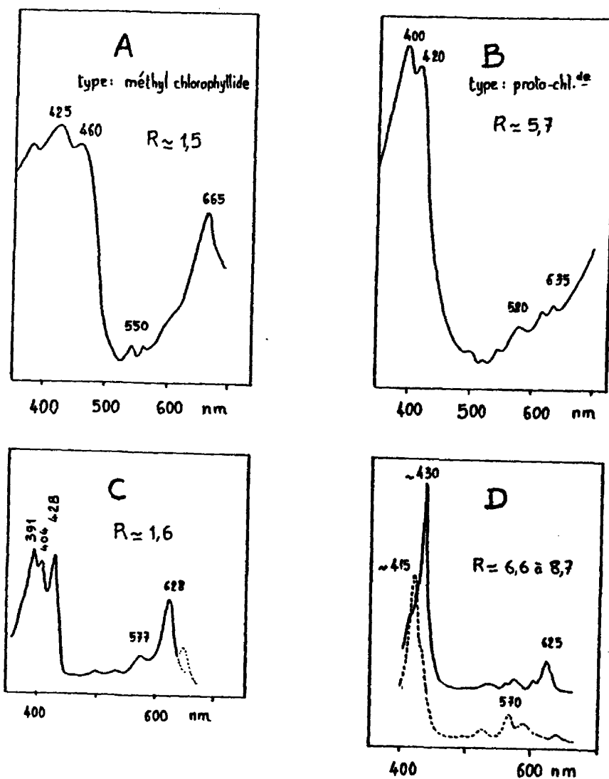
Fig. 8 - Spectres de 2 dérivés chlorophylliens de polarités élevée (A) et faible (B) comparés aux spectres dans l'éther de l'éthyl chlorophyllide (C) des protochlorophylles (D—) et des protophéophytines (D---).
